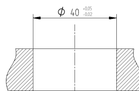
Indicazione esplicita degli scostamenti
