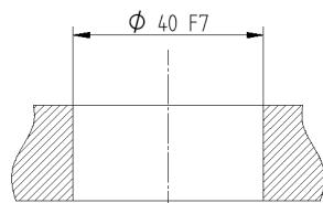
Indicazione secondo simbologia ISO
