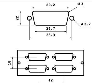
FRONTALINO INTERFACCE 24 V 15 POLI
