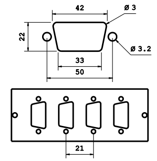
FRONTALINO INTERFACCE 24 V 9 POLI
