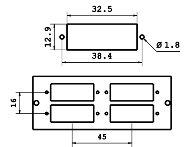
FRONTALINO ST DUPLEX 4 POS. FIBRE OTTICHE
