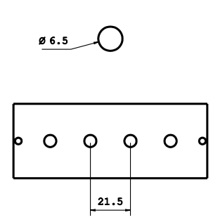
FRONTALINO F-SMA 4 POS.
