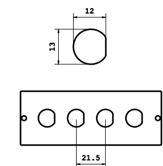
FRONTALINO BNC (tipo E) 4 POS.
