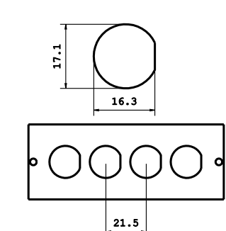
FRONTALINO BNC (tipo F) 4 POS.
