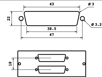
FRONTALINO INTERFACCE 24 V 25 POLI
