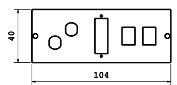
FRONTALINI CON FORATURA A RICHIESTA
