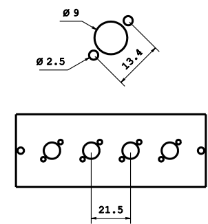
FRONTALINO FC-PC 4 POS.
