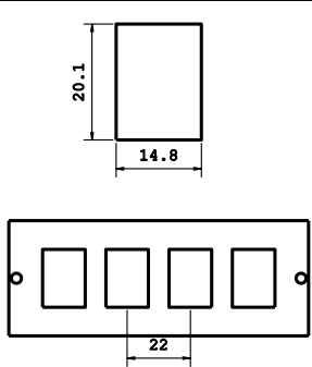
FRONTALINO RJ 4 POS.
