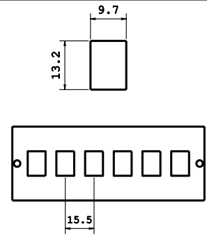
FRONTALINO SC 6 POS.
