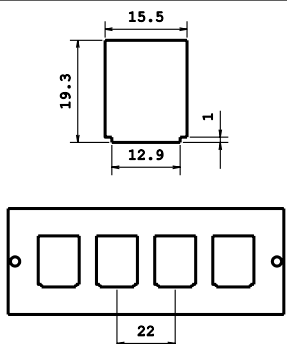
FRONTALINO RJ 11-45 4 POS.
