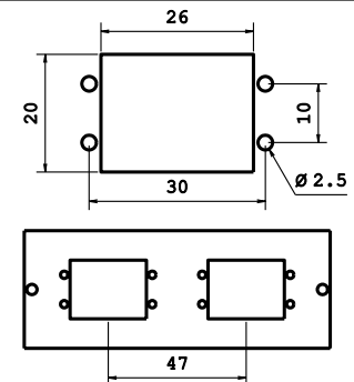
FRONTALINO SC DUPLEX 4 POS.
