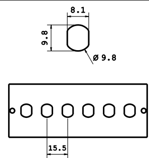
FRONTALINO ST 6 POS.
