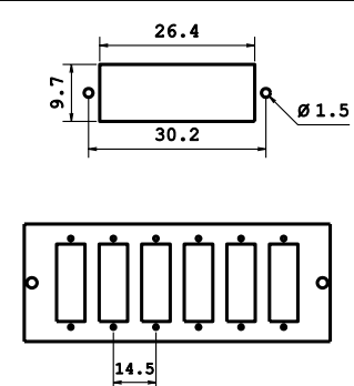
FRONTALINO SC DUPLEX 6 POS.
